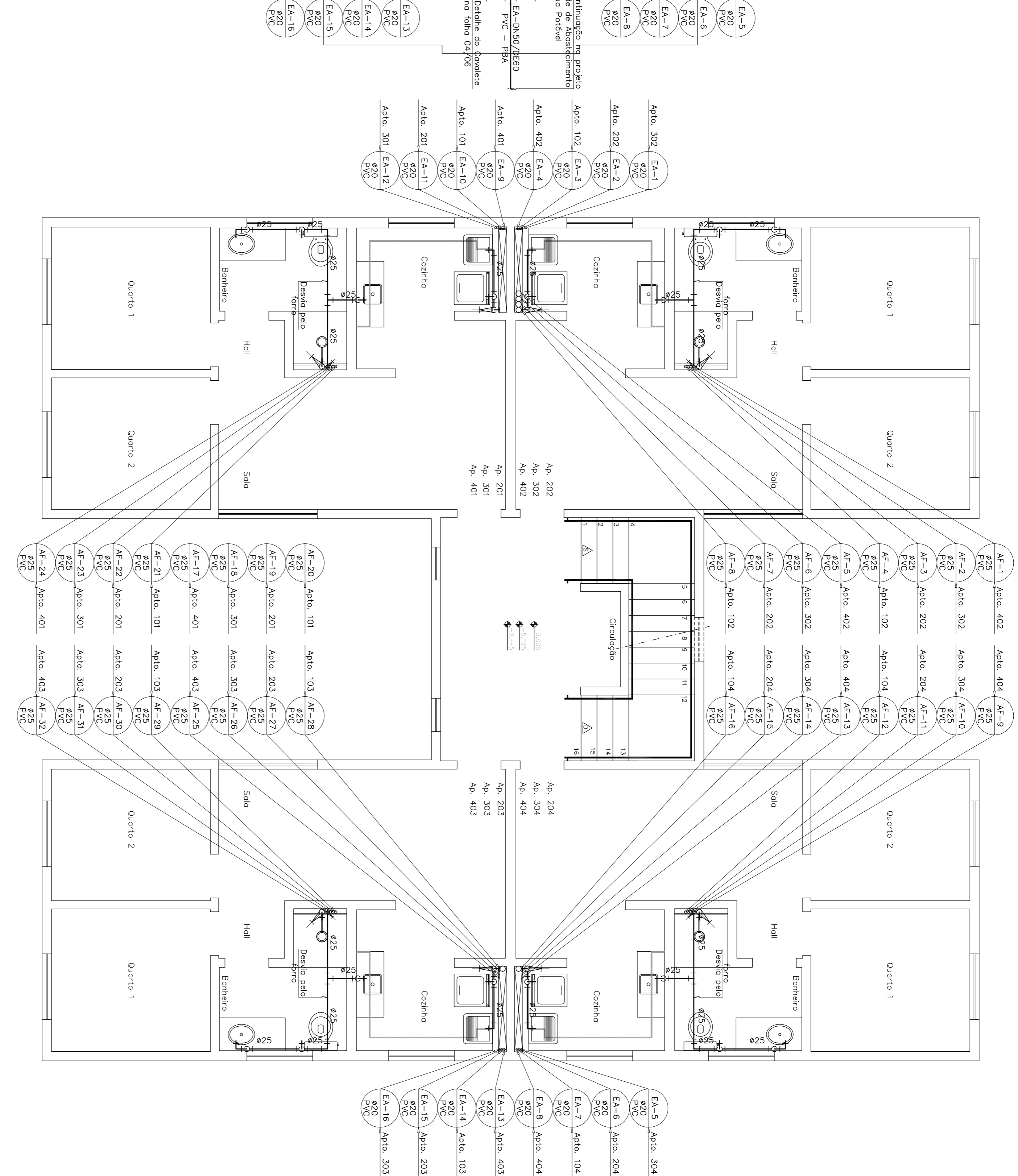
PLANTA DO PAVIMENTO TIPO – ÁGUA POTÁVEL
