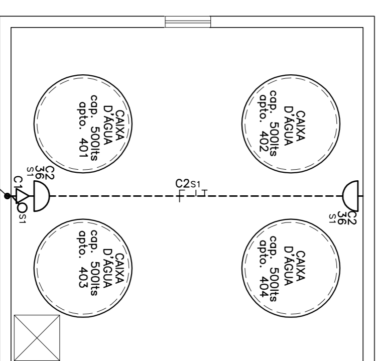
PLANTA BARRILETE ESCALA 1 : 50
